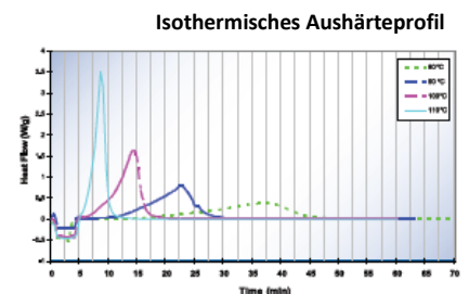
Unterschiedliche Exothermiespitzen für ein typisches Epoxy bei verschiedenen Aushärtetemperaturen
